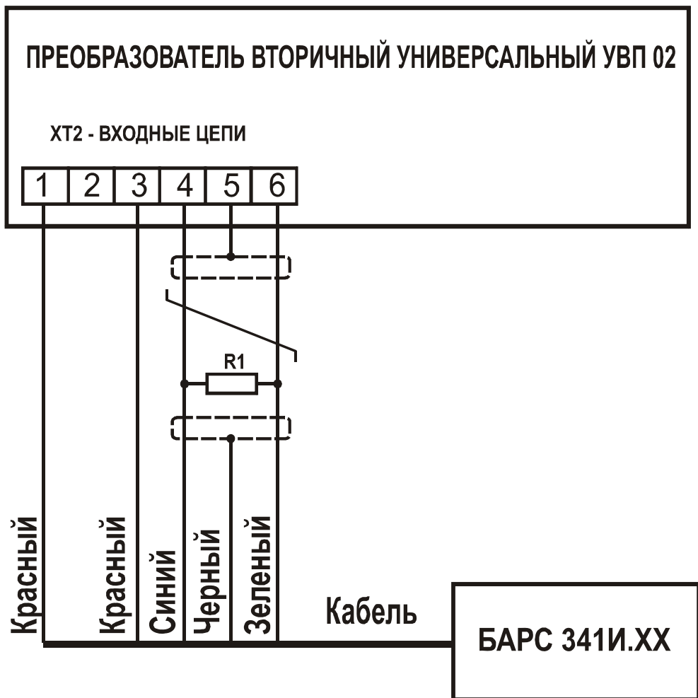
Рисунок Ж.1 – Схема электрическая подключения преобразователя уровня радиоволнового БАРС 341И.ХХ к прибору
