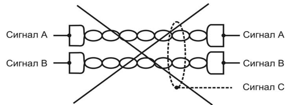
Рисунок В.7 - Неправильное подключение к витой паре
