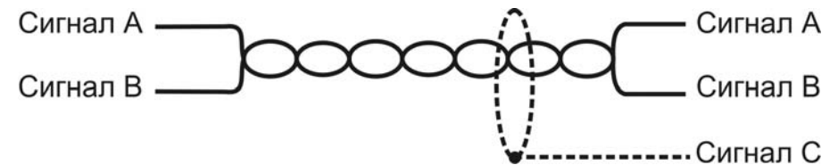
Рисунок В.6 - Правильное подключение к витой паре
