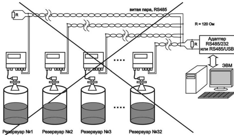
Рисунок В.5 - Неправильный монтаж витой пары на парке емкостей
