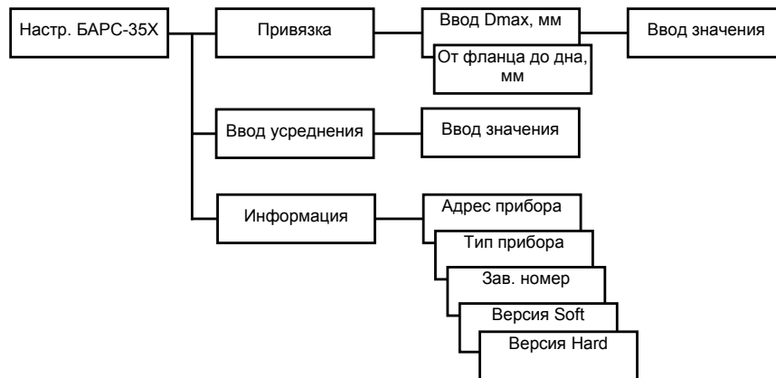
Рисунок К.2 – Меню настроек преобразователей уровня радиоволновых BARC 351И.XX и BARC 352И.XX
