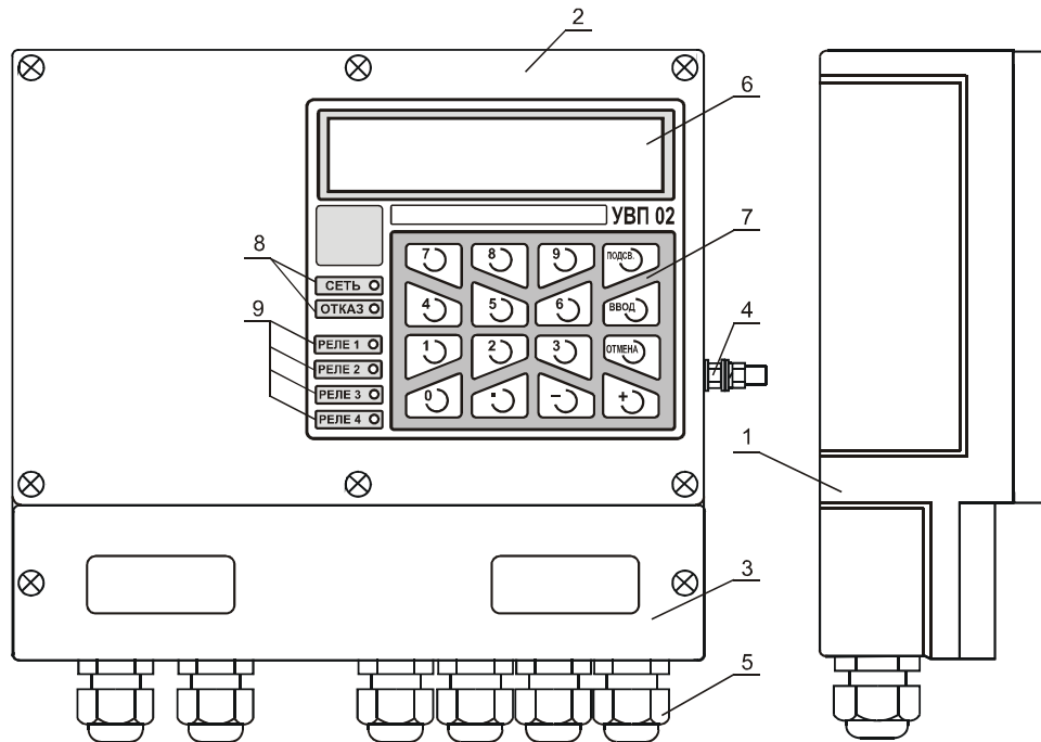
Рисунок 1 – Преобразователь вторичный универсальный УВП 02
