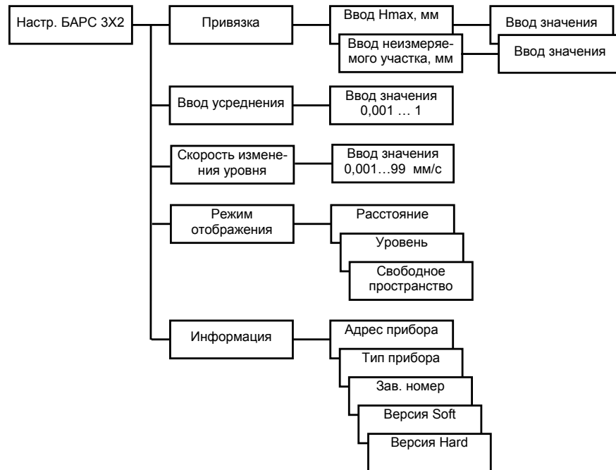
Рисунок И.2 – Схема меню настроек при работе прибора с уровнемерами радиоволновыми БАРС 322МИ-XX и БАРС 332МИ-XX
