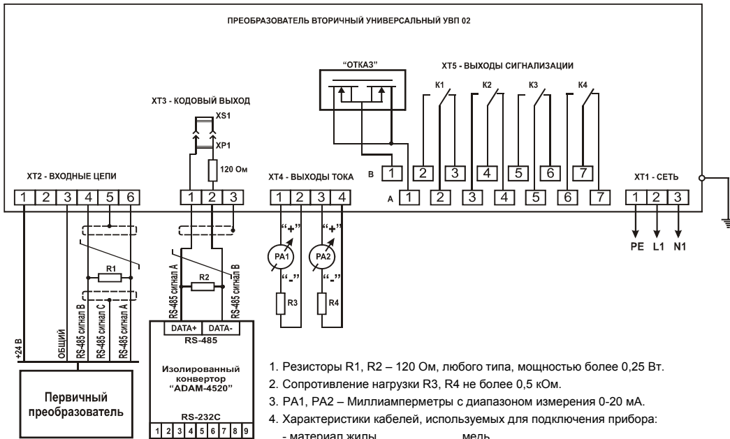
Схема электрическая подключения прибора
