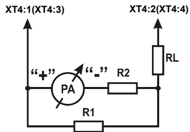
Рисунок В.2 – Подключение миллиамперметра с диапазоном измерения 0 – 5 мА
