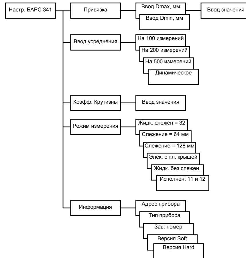
Рисунок Ж.2 – Схема меню настроек прибора при работе с преобразователем уровня радиоволновым БАРС 341И.XX
