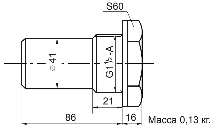
Рисунок 2 – Стакан защитный
