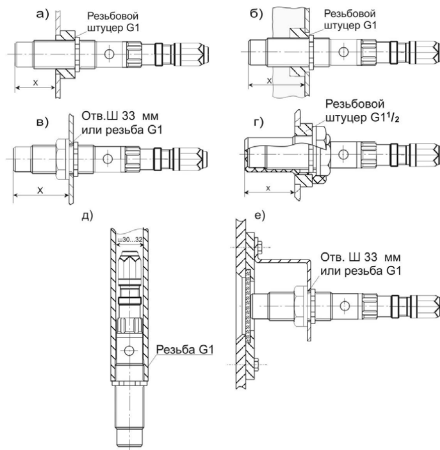
Рисунок 3 Варианты размещения сигнализатора уровня
