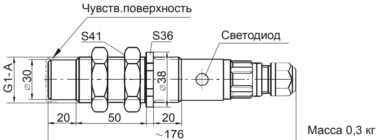
Рисунок 1 – Сигнализатор уровня
