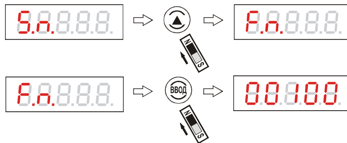
Рисунок 68 - Просмотр заводского номера урвнемера
