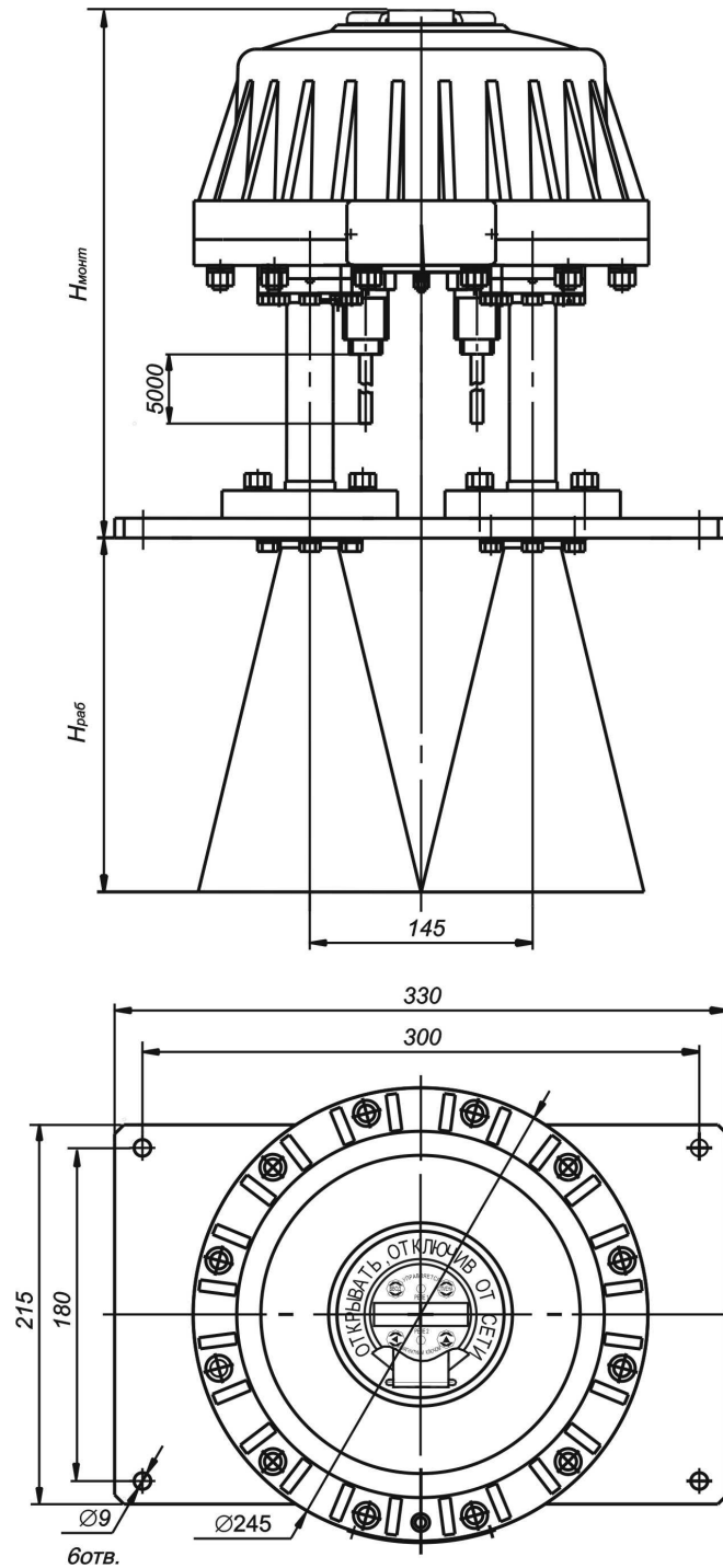
Рисунок 7 - Габаритные и установочные размеры уровня исполнения БАРС 332МИ-02
