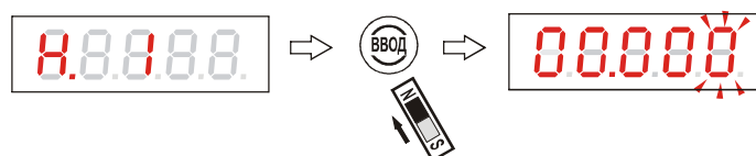
Рисунок 52 - Ввод числового значения уровня первой точки тарифовочной таблицы
