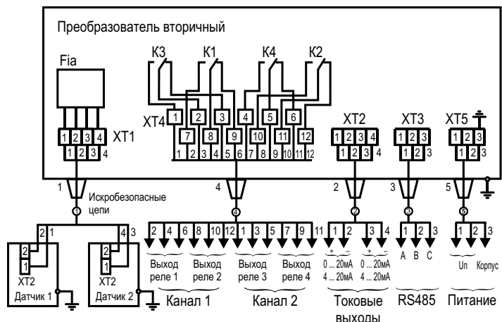
Рисунок 1 – Схема подключения
