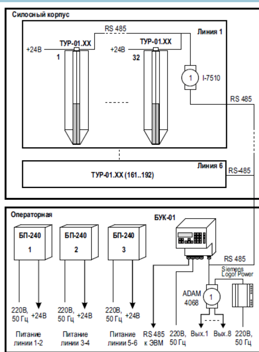
Рисунок 1 – Структурная схема АСКТ-01 с использованием термоподвесок ТУР-01
