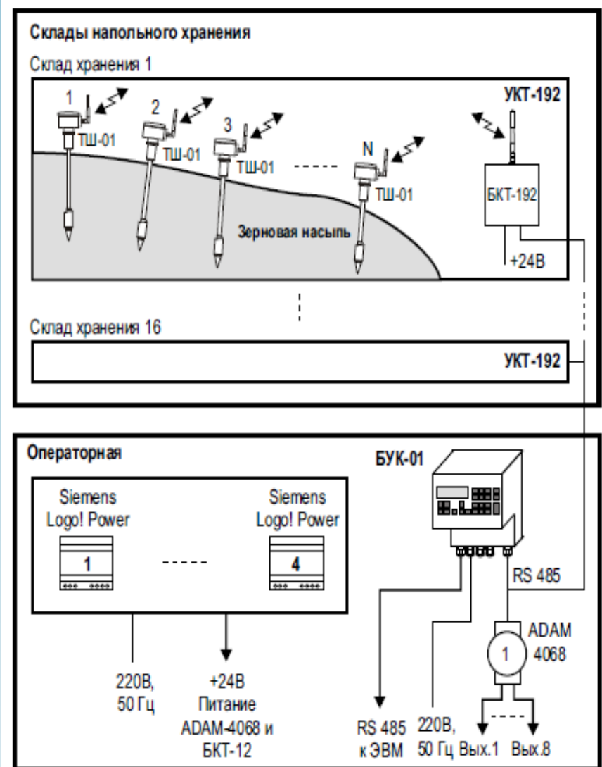
Рисунок 3 – Структурная схема АСКТ-01 с использованием термостанг ТШ-01
