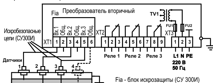
Рисунок 1 – Схема подключения
