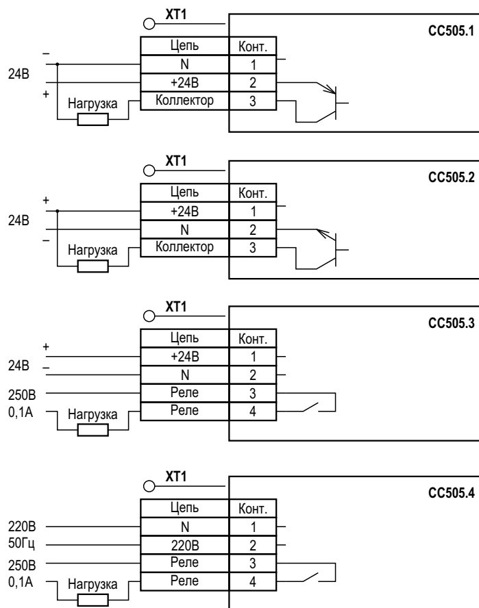
Рисунок 2 – Схемы подключения
