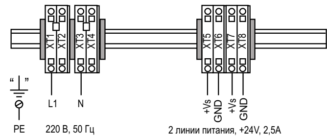
Рисунок 2 – Схема подключения блока питания БП-120
