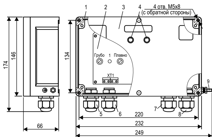
Рисунок 1 – Вторичный преобразователь
