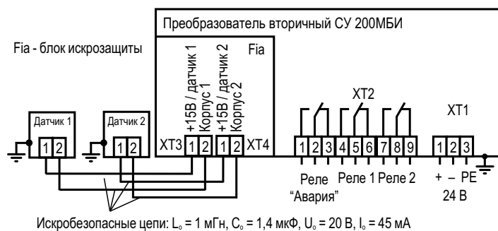
Рисунок 5 – Схема подключения сигнализатора СУ200МБИ
