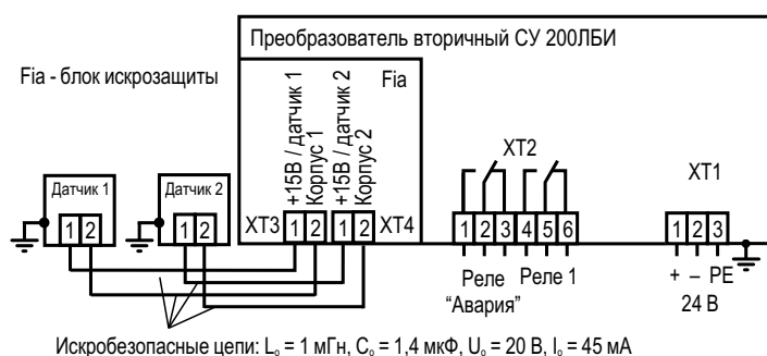
Рисунок 7 – Схема подключения сигнализатора СУ200ЛБИ
