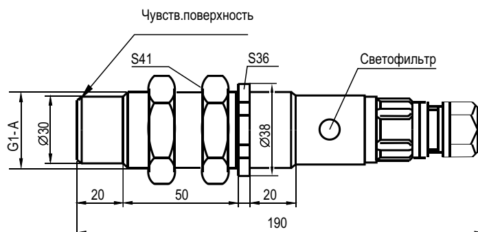
Рисунок 3 – Сигнализатор скорости CC505
