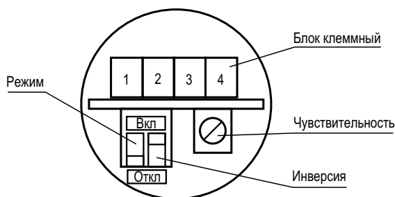
Рисунок 1 – Монтажная зона сигнализатора CC505
