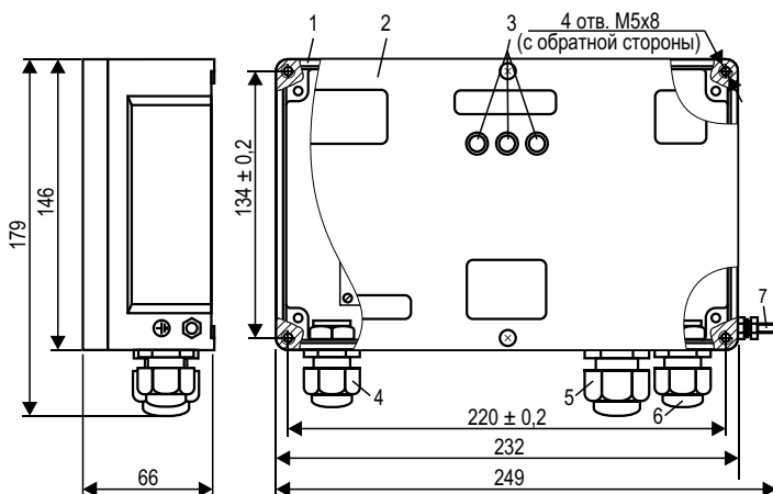
Рисунок 4 – Вторичный преобразователь
