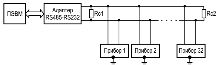
Рисунок 3 – Схема подключения ТЕМП-01 к линии связи RS-485
