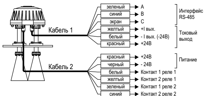
Рисунок 3 – Схема подключения
