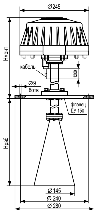
Рисунок 2 БАРС341И.03 – БАРС341И.05
