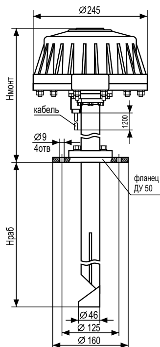
Рисунок 7 БАРС351И.18
