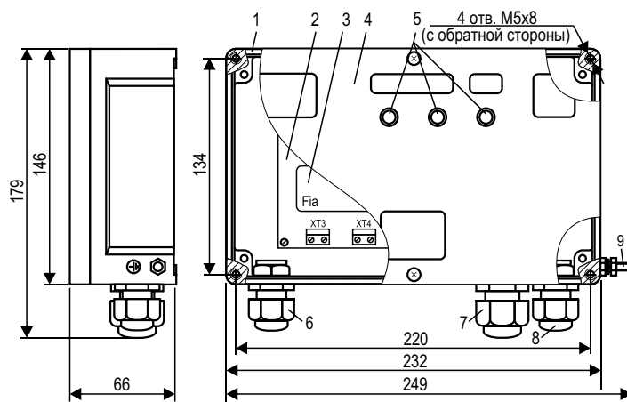
Рисунок 3 – Вторичный преобразователь СУ200ЛАИ, СУ200ЛБИ
