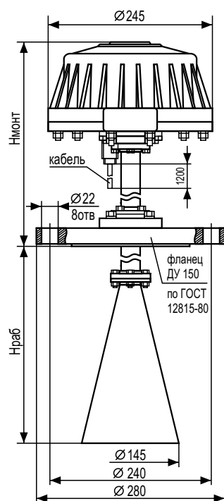
Рисунок 3 БАРС341И.06 – БАРС341И.08
