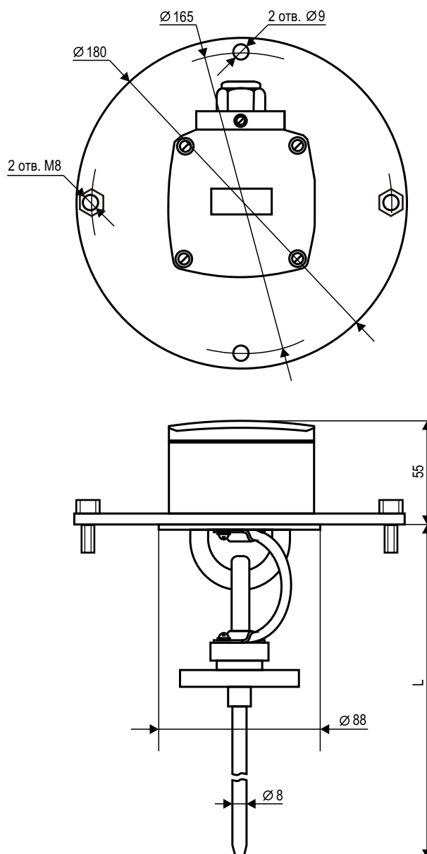
Рисунок 3 – Термоподвеска ТП-01.XX
