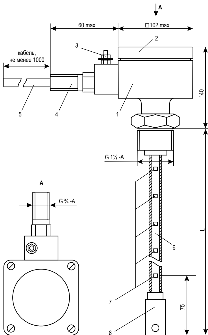
Рисунок 2 – Преобразователь температуры ТЕМП-01
