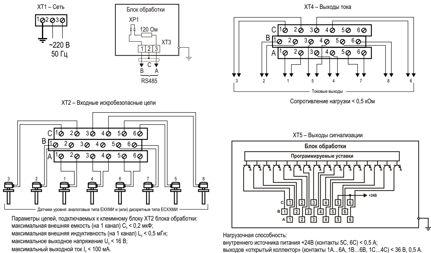
Рисунок 2 – Схема подключения
