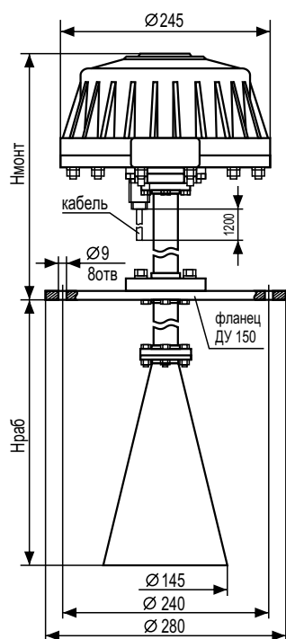
Рисунок 2 БАРС351И.00 – БАРС351И.04
