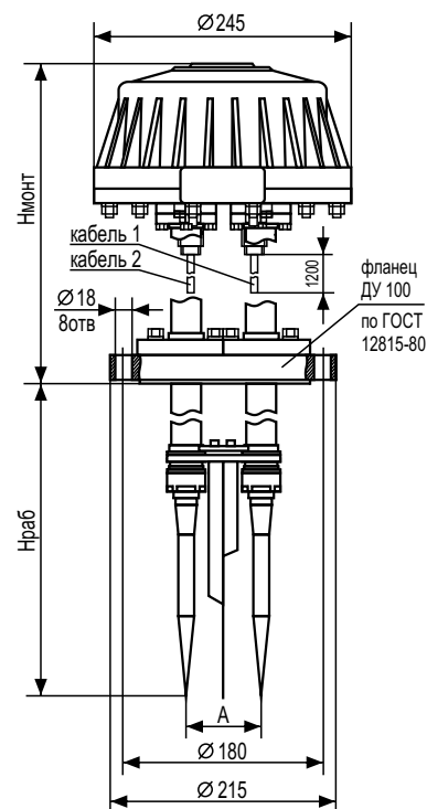
Рисунок 2 – БАРС 322МИ-07
