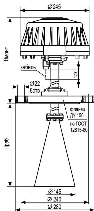
Рисунок 3 БАРС351И.06 – БАРС351И.10
