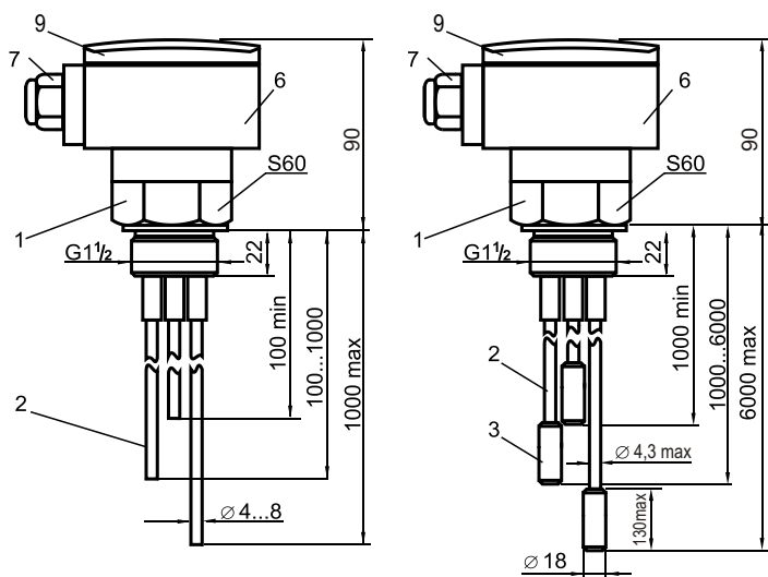
Рисунок 3 – Трехэлектродные датчики
