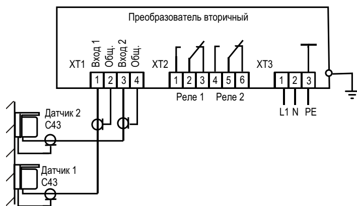
Рисунок 3 – Схема подключения
