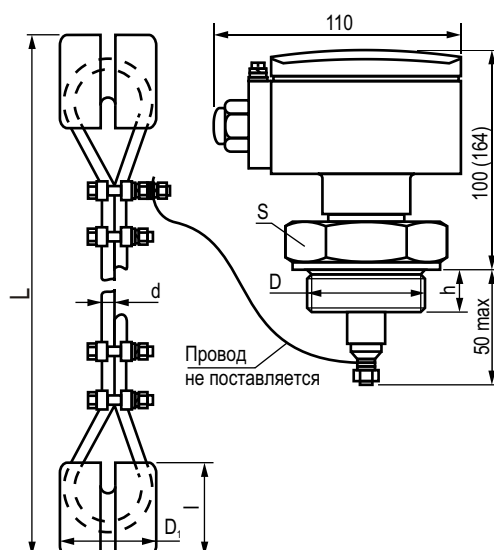
Рисунок 6 – Сигнализаторы с тросовыми ЧЭ
