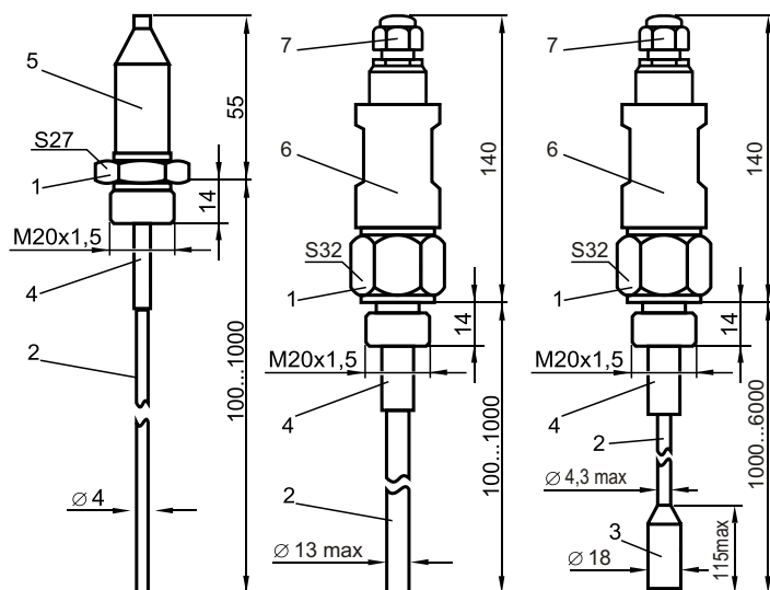
Рисунок 2 – Одноэлектродные датчики
