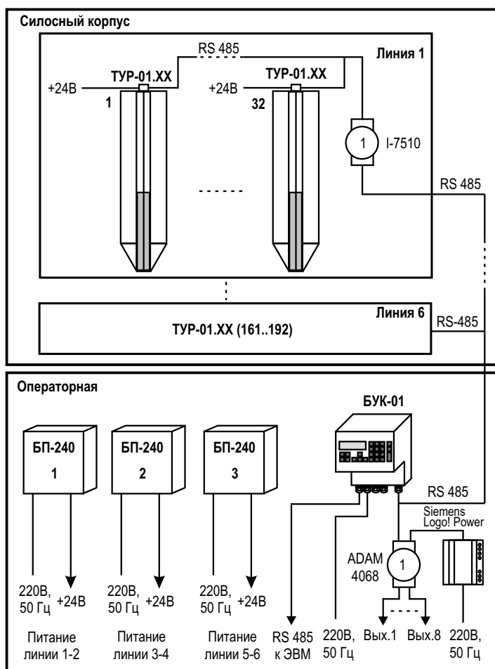
Рисунок 1 – Структурная схема АСКТ-01 с использованием термоподвесок ТУР-01
