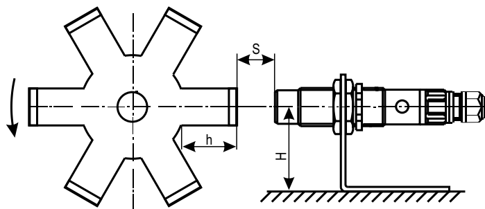
Рисунок 4 – Монтаж сигнализатора
